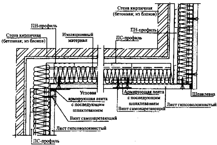
Б Т-сопряжение
