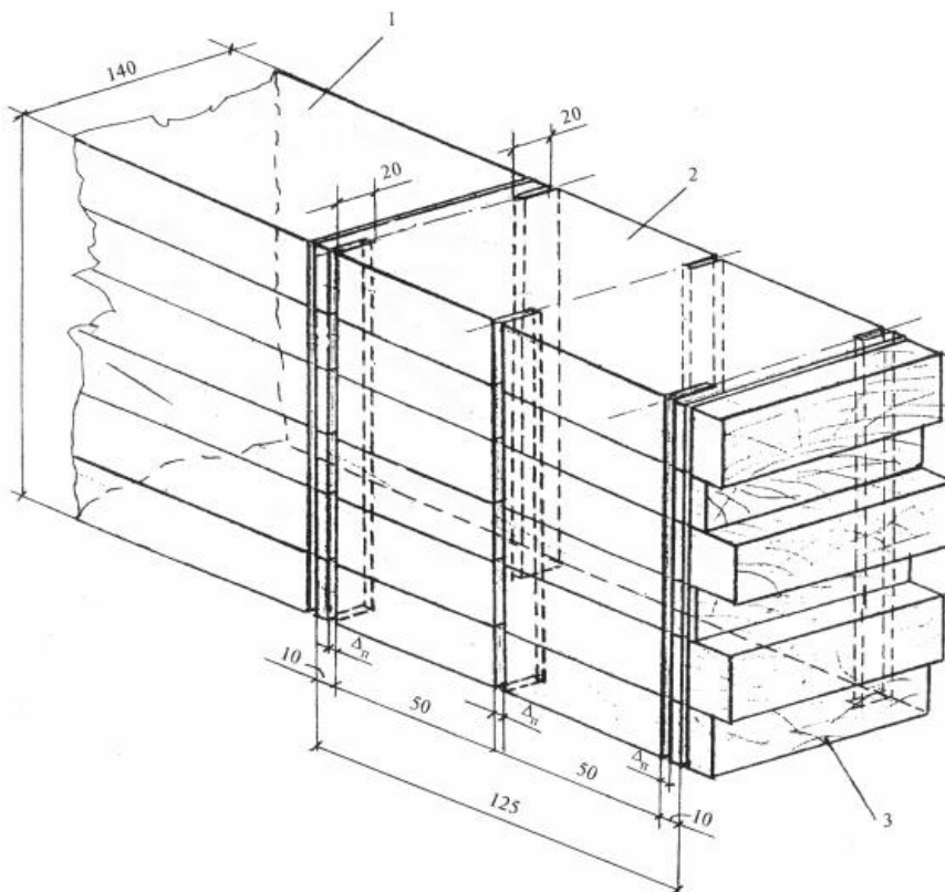
1 - клееный элемент; 2 - образец для испытаний; 3 - отпад при торцовке элемента; \Delta_n - ширина пропила
