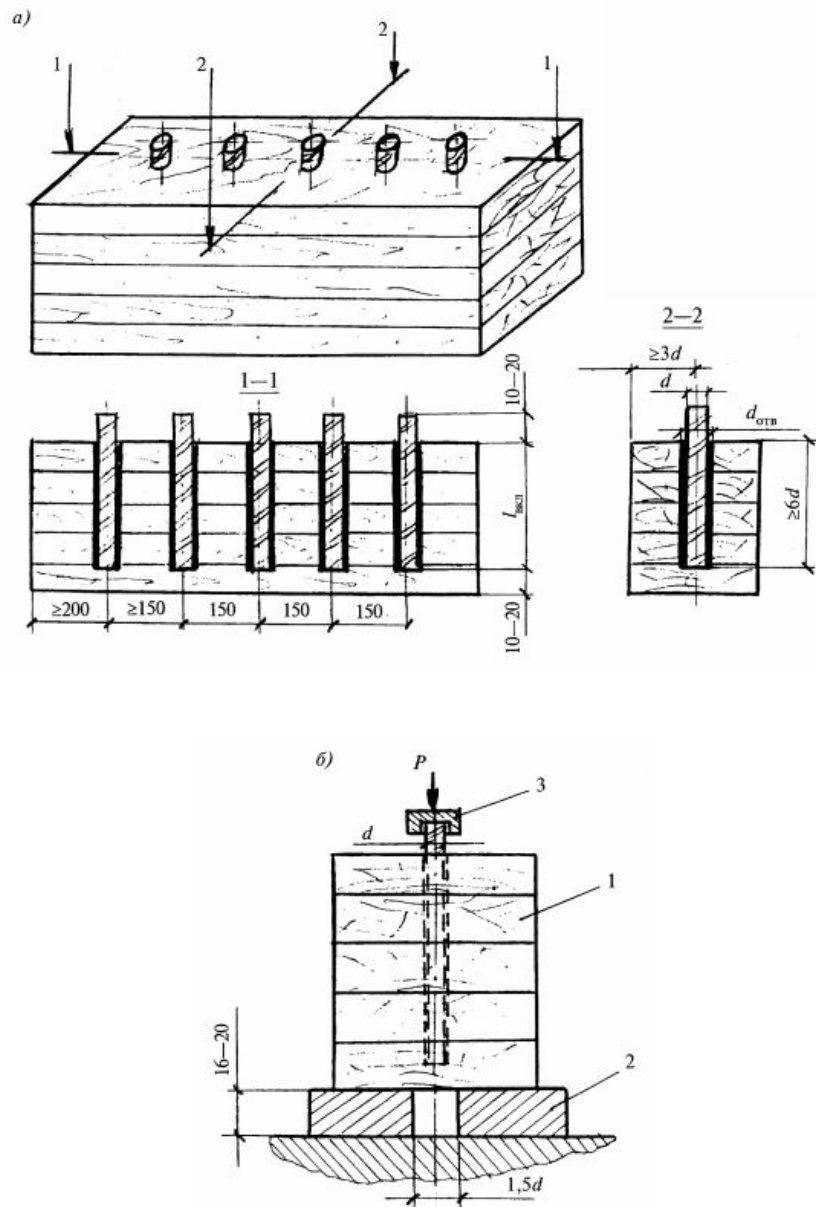
а - заготовка с вклеенными стержнями; б - схема испытаний; 1 - древесина; 2 - металлическая подкладка с отверстием; 3 - металлический шарнир
