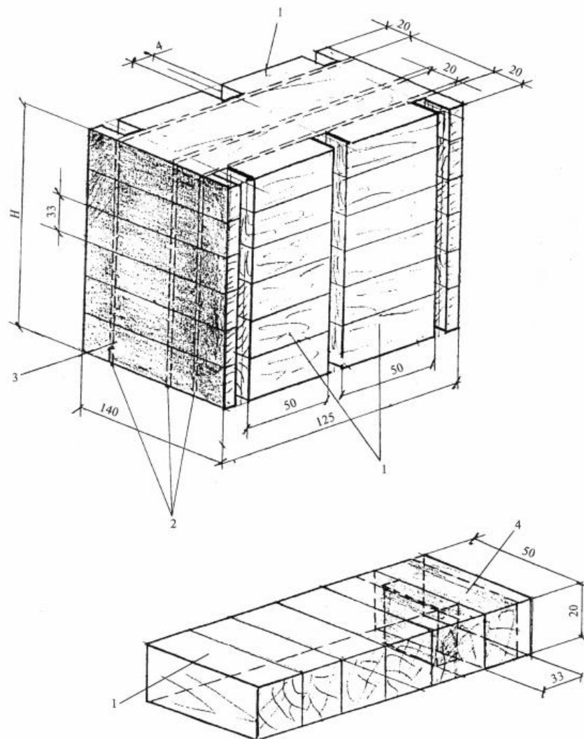
1 - заготовка для выпиливания образцов для испытаний на скалывание по ГОСТ 15613.1; 2 - пропилы при выпиливании заготовок; 3 - торцы образцов (перед вымачиванием покрыть эпоксидной шпатлевкой ЭП-001); 4 - образец для испытаний на скалывание по ГОСТ 15613.1
