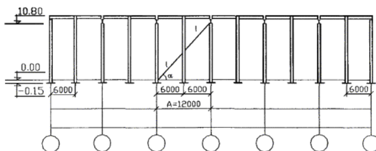
Крепление связей на болтах
