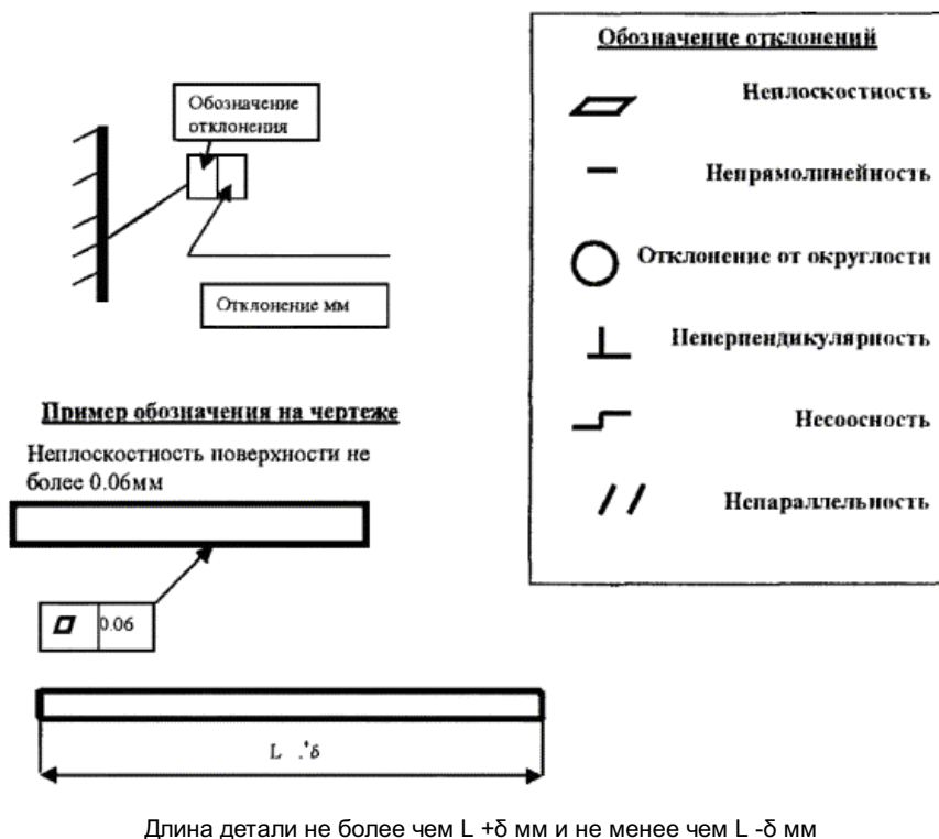
Рисунок 3 - Обозначение на чертежах предельных отклонений размеров и формы элемента
