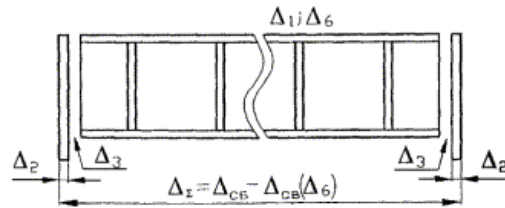
Рис. 2 Схема балки
