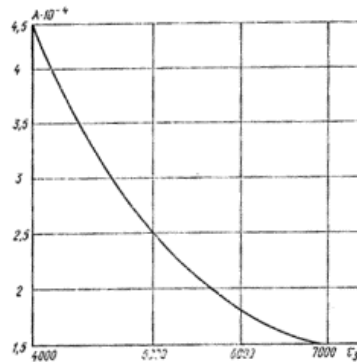
Рис. 33. Номограмма для определения значения A
