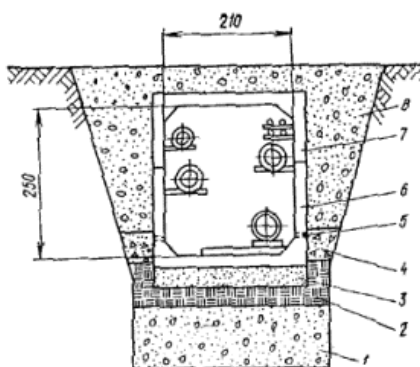
Рис. 10. Конструкция канала на просадочных при оттаивании грунтах
