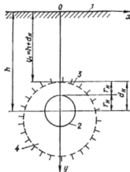
Рис. 43. Схема для расчета талика вокруг трубопровода
