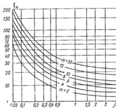
Рис. 39. Номограмма для определения коэффициента x_n
