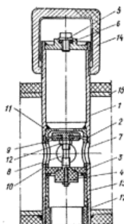
Рис. 21. Автоматический выпуск воды
