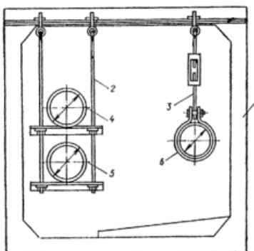
Рис. 16. Прокладка трубопроводов на подвесках в канале
