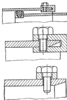
Рис. 26. Самоуплотняющийся компенсатор для воды с устройством против разрыва
