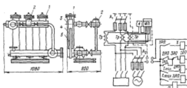
Рис. 18. Электродный котел
