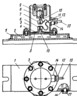
Рис. 20. Конструкция терморегулятора
