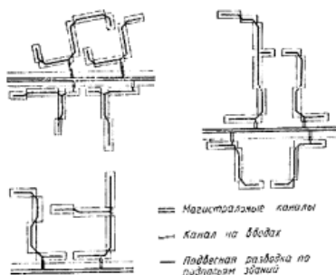
Рис. 13. Вводы в здание
