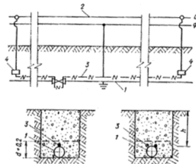
Рис. 19. Схема оборудования водопровода греющим кабелем
