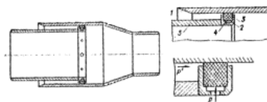
Рис. 23. Самоуплотняющийся компенсатор для воды
