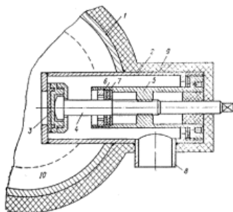
Рис. 28. Конструкция выпуска воды при оледенении трубопровода на 50 %
