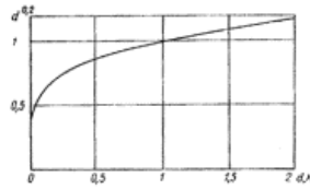
Рис. 37. График для определения величины x
