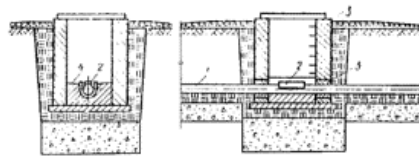
Рис. 30. Смотровой колодец на сети канализации, оборудованный закрытой ревизией с клиновым уплотнением крышки
