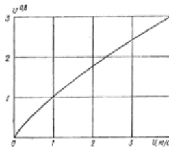
Рис. 36. График для определения величины \sqrt{0,8}
