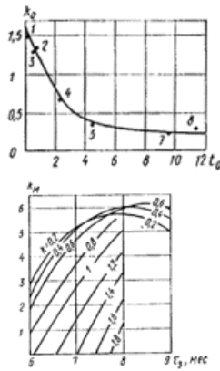
Рис. 35. Номограмма для определения вспомогательных величин K_0, K_M, h
