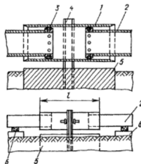
Рис. 24. Двусторонний самоуплотняющийся компенсатор для воды
