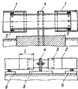
Рис. 25. Двусторонний самоуплотняющийся компенсатор для воды
