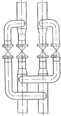
Рис. 31. Узел переключений с перекрестными перемычками
