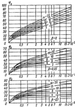
Рис. 41. Номограмма для определения коэффициента \beta_0
