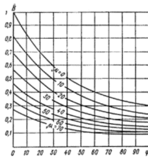
Рис. 34. Номограмма для определения значения B
