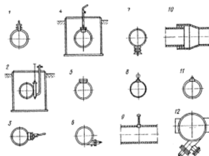
Рис. 27. Установка незамерзающей арматуры на водопроводе
