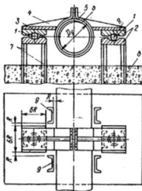
Рис. 14. Конструкция шаровой опоры
