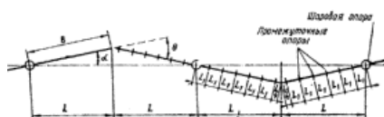
Рис. 15. Прокладка трубопровода на шаровых и скользящих опорах
