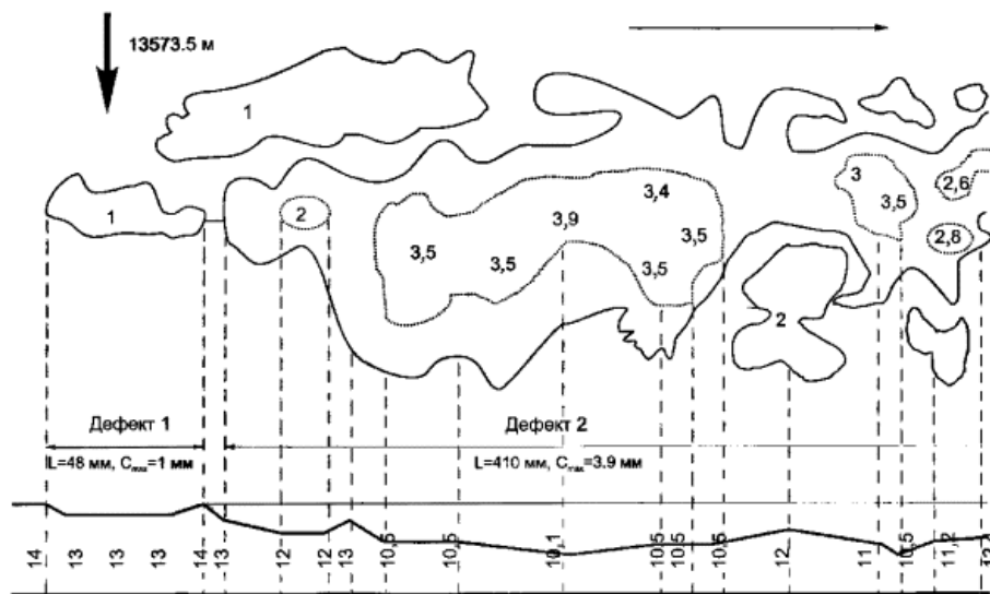
Рис. 3 Схема коррозионных повреждений наружной поверхности газопровода (фрагмент)
